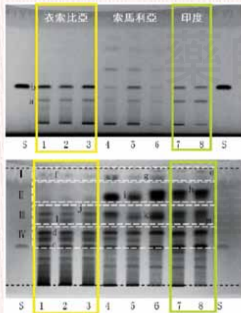
(a) 11-羧基-β-乳香酸 (b) 11-羧基-β-乙酰乳香酸 (c) α,β-乳香脂酸 (d) α,β-乙酰乳香酸
