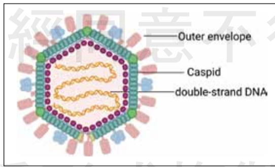
↑圖一 2 病毒結構。
